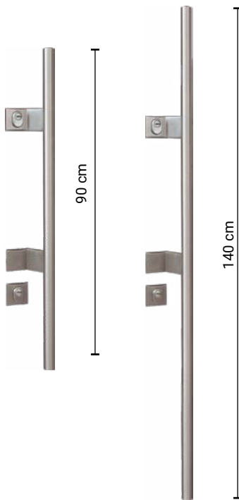
A2 INOX 90cm kerek ajtóhúzó (belső oldalon Tamara kilinccsel)
