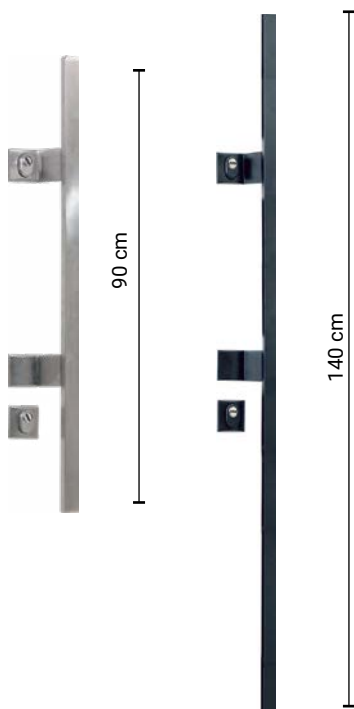
A2 INOX 90cm szögletes ajtóhúzó (belső oldalon Tamara kilinccsel)
