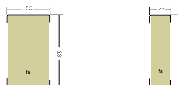
Termo ODS toktoldók
