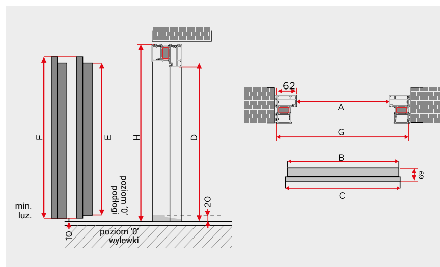
SPECIAL és MASTER ajtószárnyak méretei
