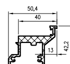
DRE profil pre dovnútra otvárateľné reverzné falcové dvere
