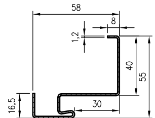
OSMK door frame profile
