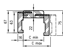
Prierez TUN s uhl. T63
