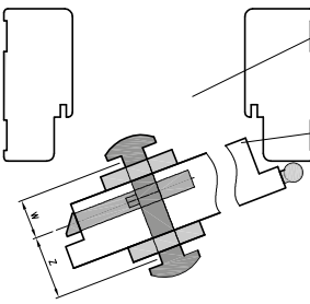
Obr. Výber veľkosti vložky s gombíkom
