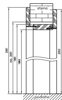
Vertikálna časť nastaviteľného tunelu s uhl. T80
