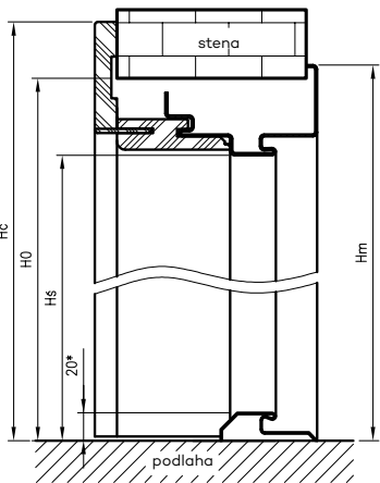
Rozmery OSH STAND pre dvojkrídlové dvere
