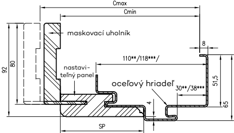
Profil zárubne
