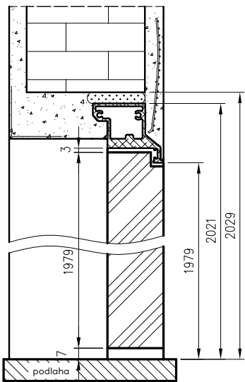
DRE profil pre dovnútra otvá- teľné reverzné falcové dvere
