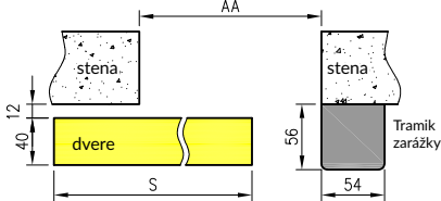
NS - horizontálny prierez (ľavý systém)
