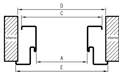
D - šírka montážneho otvoru
