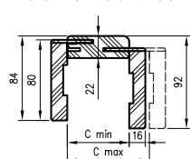
Prierez TUN s uhl. T63
