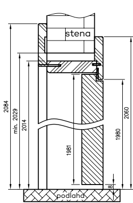
Vertikálny prierez ORO
