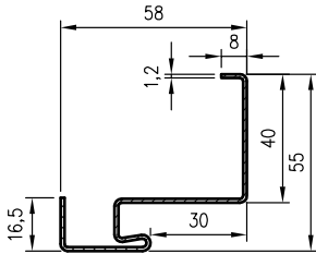
Profil zárubne OSMK
