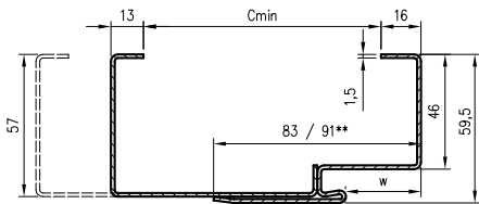
Profil zárubne s uzatváracím uholníkom T57
