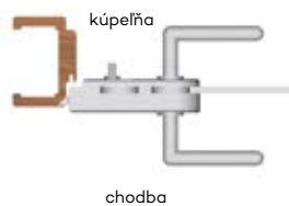
obr. 3. pravé dvere / vnútorný zámok
