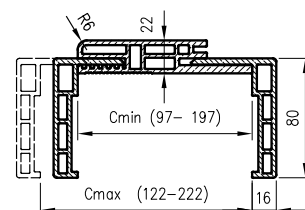
Przekrój belki ORB Water Proof dla Cmin 97-197 mm
