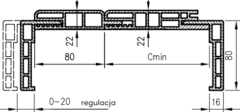
Przekrój belki OR Water Proof + panel OR Water Proof o szerokości 200-260 mm
