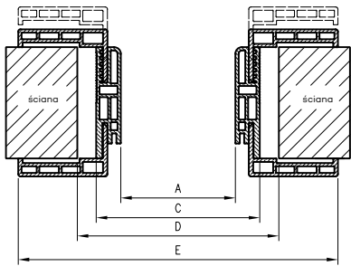
Przekrój poziomy OR Water Proof
