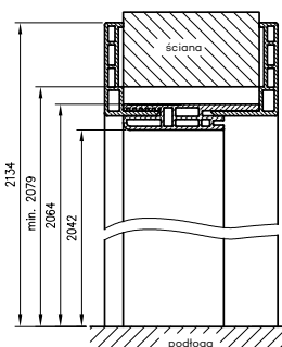
Przekrój pionowy ORB Water Proof
