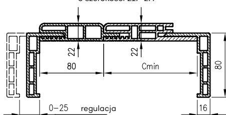
Przekrój belki ORB Water Proof + panel ORB Water Proof o szerokości 217-277
