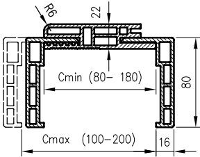
Przekrój belki OR Water Proof o szerokości 80-180 mm
