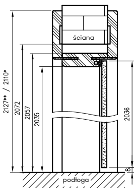
Przekrój pionowy drzwi szklanych z ORC
