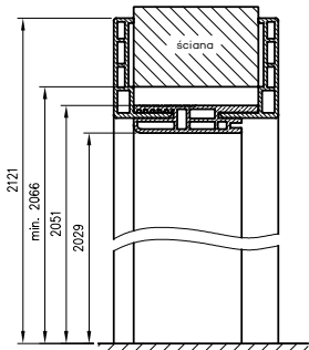
Przekrój pionowy OR Water Proof
