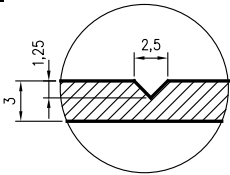
szkic frezu "V"
