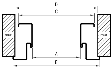
D - szerokość otworu montażowego
