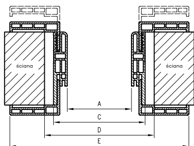
Przekrój poziomy ORB Water Proof
